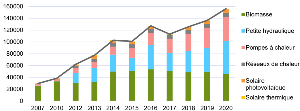
Production d'énergie sur le territoire (MWh/an)
